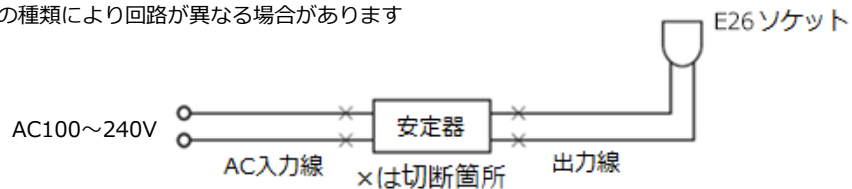
図①：現行の配線と切断箇所
